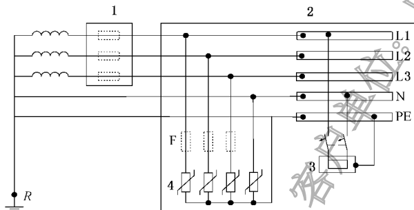
图 E.1 TN-C-S 系统中在进户处电涌保护器的安装示例
